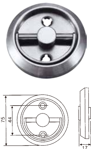
K2928-1 圓盤拉手
