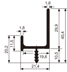
A446 (適用6分板)
