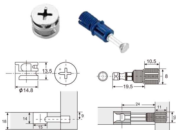
M3081 KD組合螺絲
