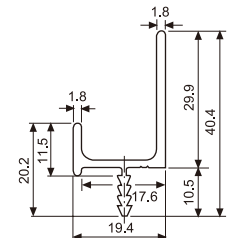
A446-1 (適用6分木芯板 長度為訂製品)
