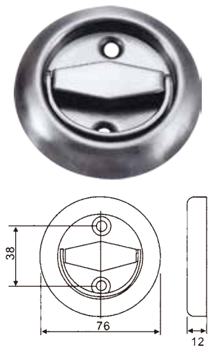
K2928-2 圓盤拉手
