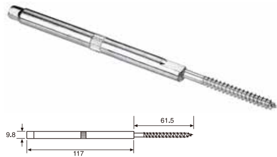
M3080 固格組合螺絲 \phi 3mm
