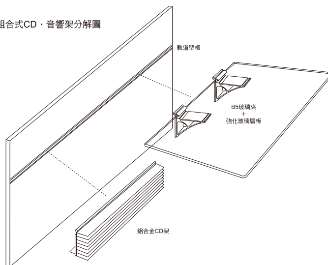
B5 軌道配件
