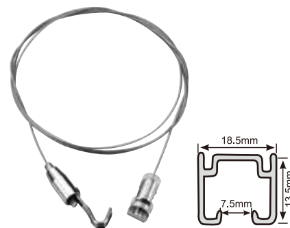
658 快拆型吊圖鋼索掛勾 (5尺)
