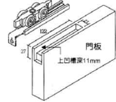
2. 隱藏式安裝法
