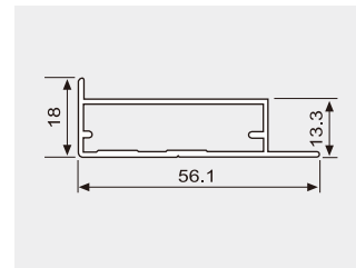
後面可夾12mm木板
