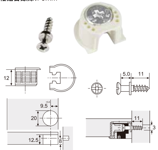
M3080 固格組合螺絲 \phi 3mm
