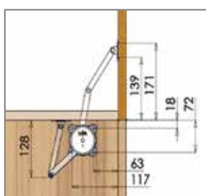
I3052 SUSPA 櫃體安全緩衝撐桿
