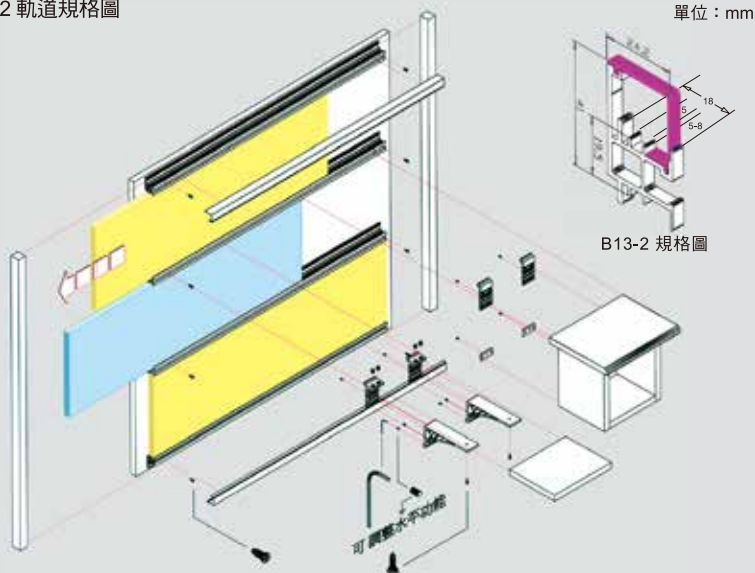
B13-2 軌道規格圖
