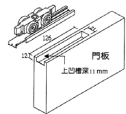
2. 隱藏式安裝法
