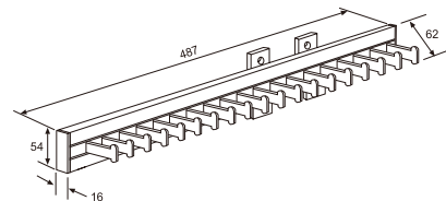
L13B 領帶架(皮帶架)
